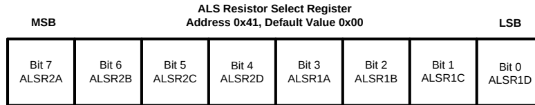
Figure 45. ALS Resistor Select Register
