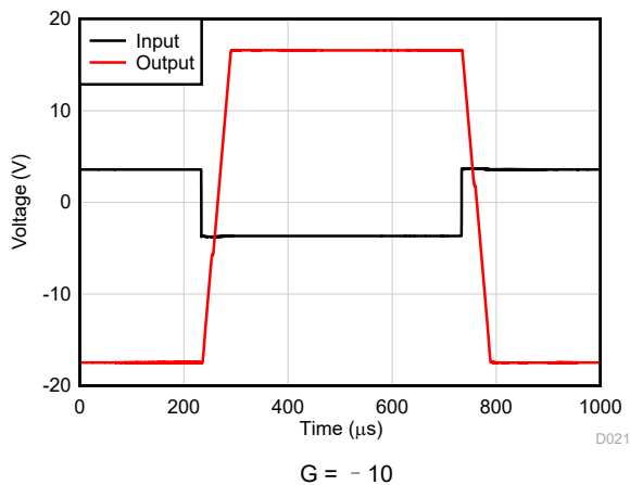
图 6-28. Overload Recovery
