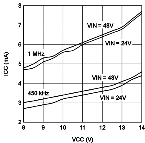
图 6-4. I_{CC} vs External V_{CC}
