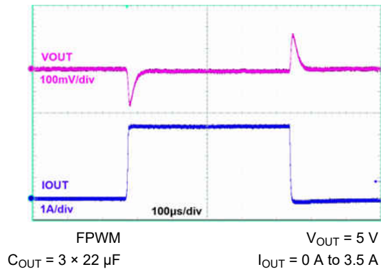
图 9-17. Load Transient
