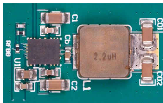
典型车用布局 (22mm x 12.5mm)
