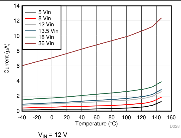
图 7-6. Shutdown Current
