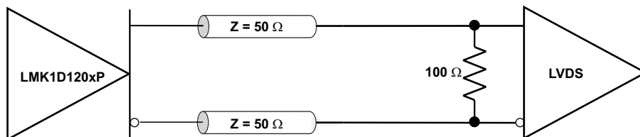
图 8-1. Output DC Termination
