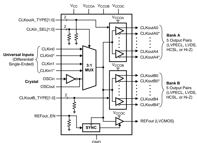
功能框图
