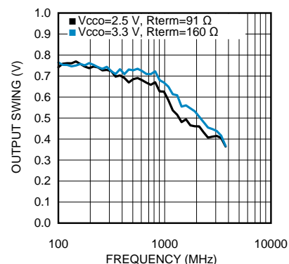
LVPECL 输出摆幅 (V OD ) 与频率间的关系
