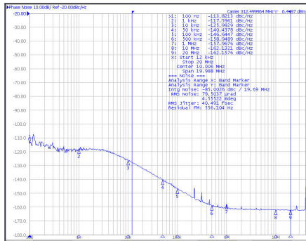
图 9-4. 312.5 MHz Output Phase Noise (APLL3 BAW)
