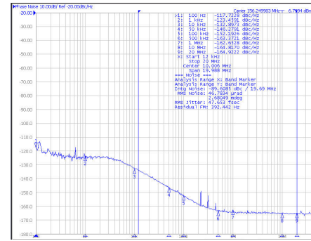
图 9-5. 156.25-MHz Output Phase Noise (APLL3 BAW)
