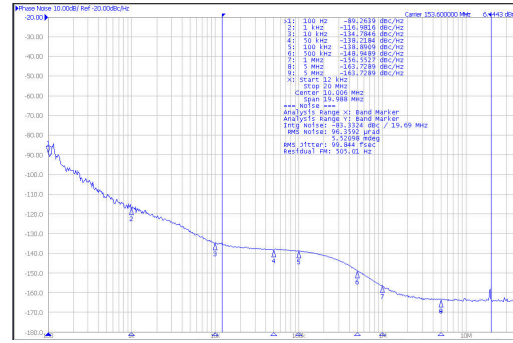
图 9-11. 153.6 MHz Output Phase Noise (APLL2)
