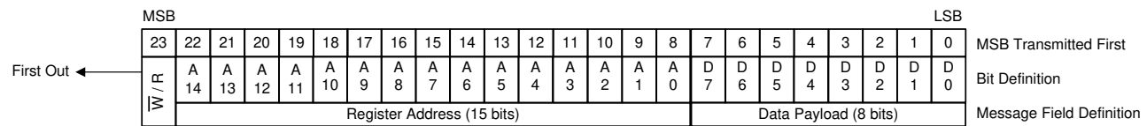
图 8-42. SPI Message Format
