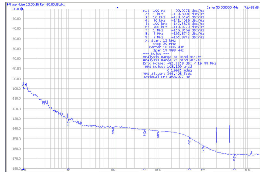
图 9-16. 50-MHz Output Phase Noise (APLL1)
