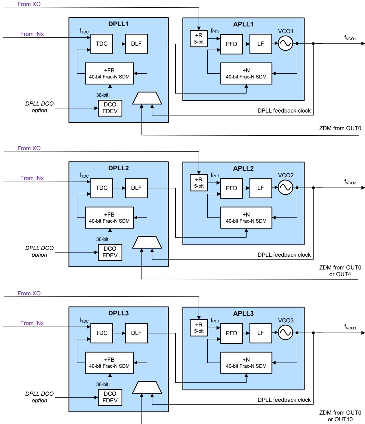
图 8-3. DPLL Independent Mode
