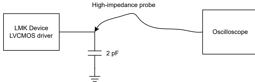
图 7-3. LVC MOS Output Time Domain Test Configuration
