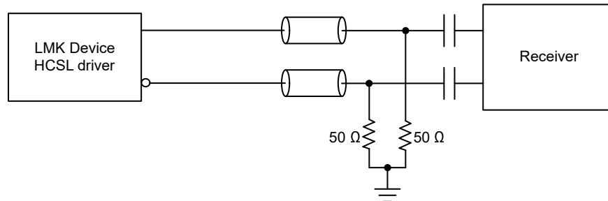
图 8-28. AC-Coupled HCSL Output Termination
