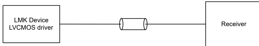
图 8-23. LVCMOS Output Termination
