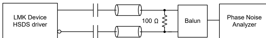
图 7-6. HSDS Output Phase Domain Test Configuration
