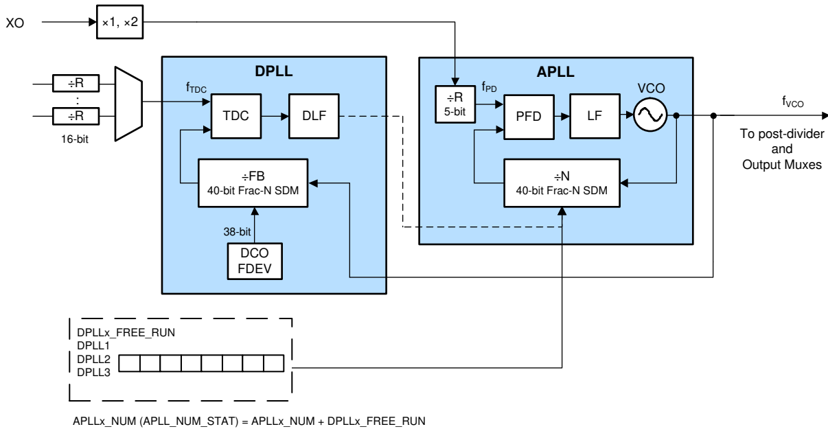
图 8-39. APLL DCO Mode
