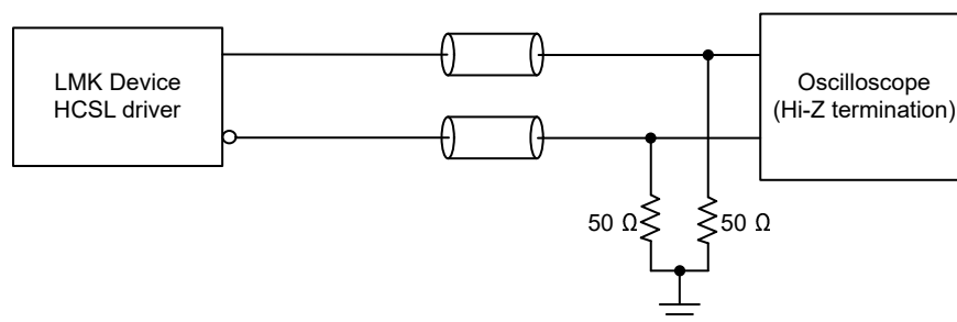
图 7-7. HCSL Output Time Domain Test Configuration
