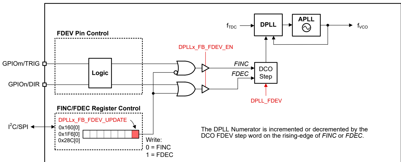
图 8-38. DCO Mode Control Options
