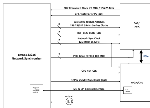
LMK5B33216 典型系统方框图
