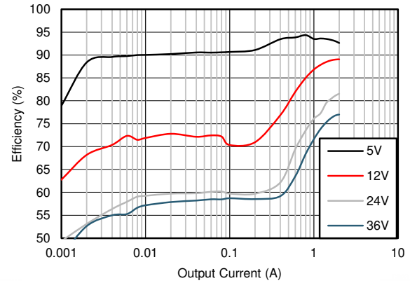
图 8-16. Efficiency
