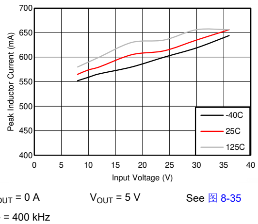
图 6-6. I_{PEAK-MIN}
