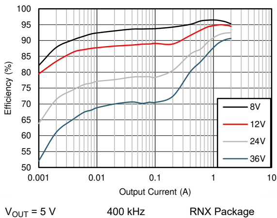
图 8-11. Efficiency
