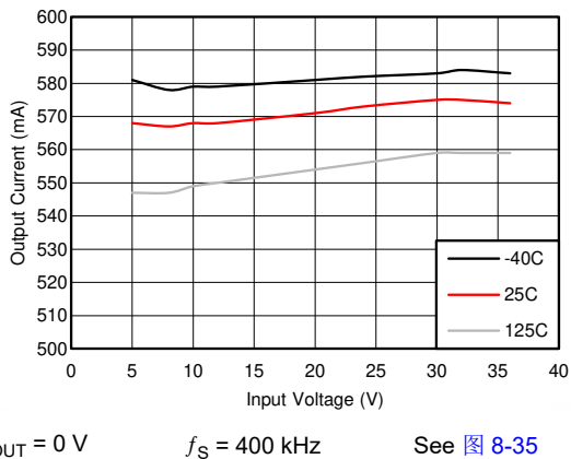
图 6-3. Short-Circuit Output Current
