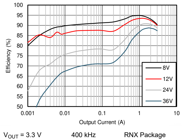
图 8-10. Efficiency
