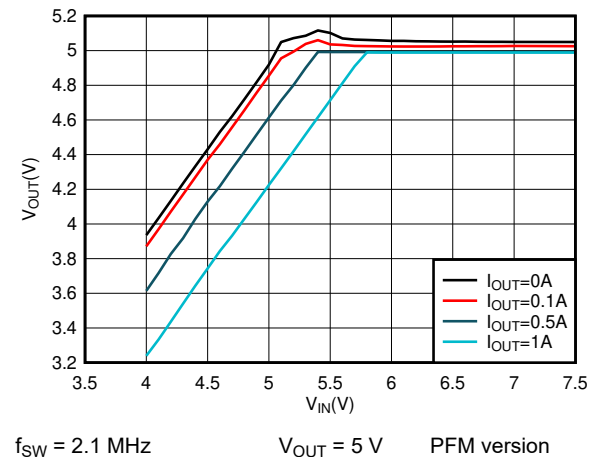
图 7-5. 5-V Dropout
