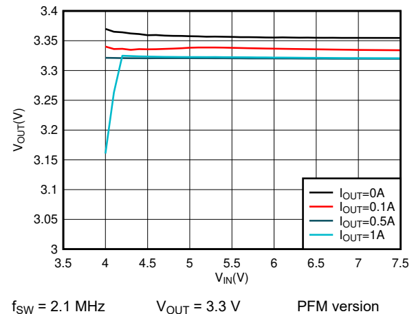
图 7-6. 3.3-V Dropout
