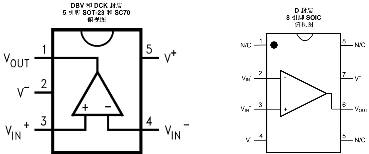
引脚功能
