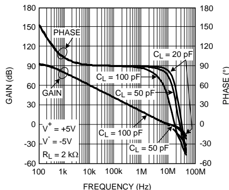
图 14. 带容性负载的开环增益和相位
