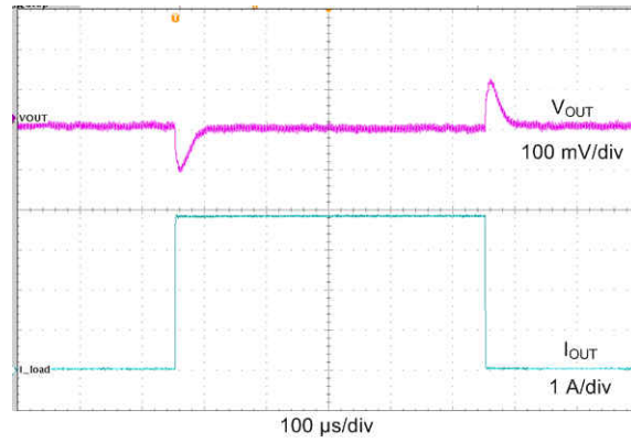
图 9-33. Load Transient
