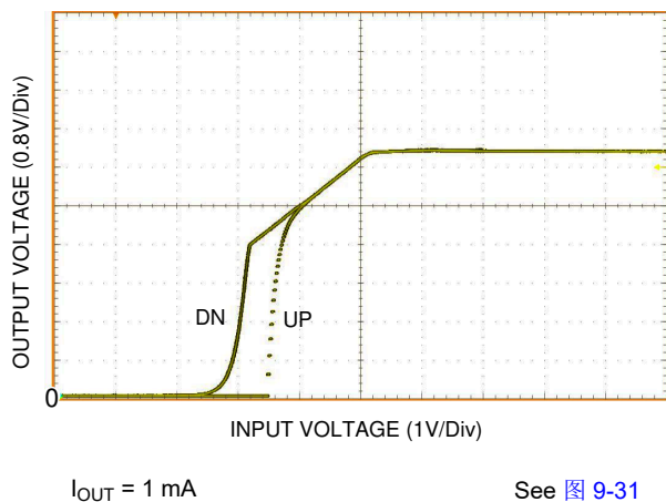
图 7-5. UVLO Thresholds
