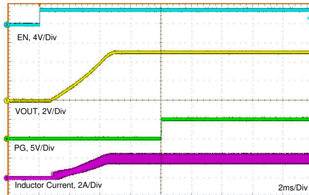
图 8-3. Precision Enable Behavior
