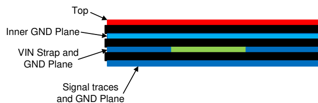
图 10-3. Example Layout for VQFN Package
