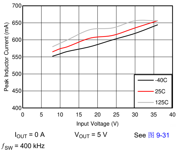
图 7-6. I_{PEAK-MIN}
