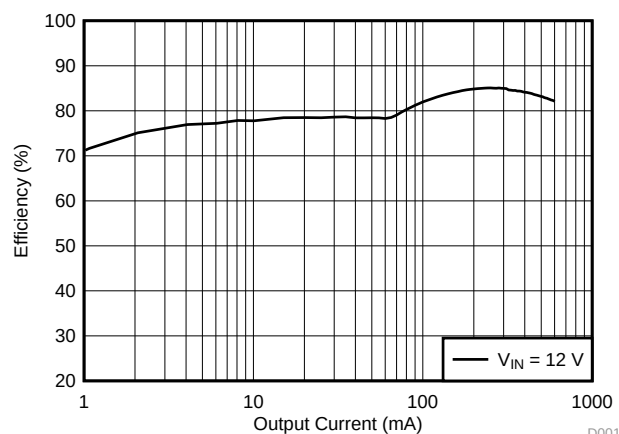
效率与输出电流间的关系 ( f_{\text{SW}} = 2.1\text{MHz} , V_{\text{OUT}} = 3.3\text{V} )
