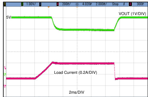
图 8-16. Overload Output Recovery
