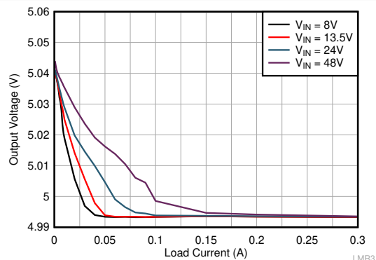
LMR36503MSC5 V_{OUT} = 5 V Fixed 2.2 MHz (AUTO)
