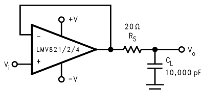
图 36. 使用隔离电阻器来驱动大型容性负载
