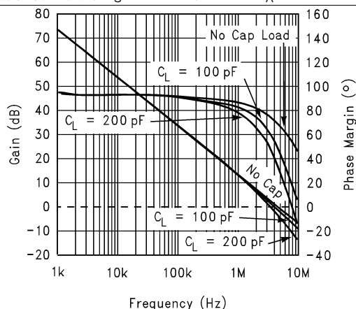
图 25. 增益和相位裕度与频率间的关系 ( C_L = 100\text{ pF} , 200\text{ pF} , 0\text{ pF} , R_L = 600\text{ }\Omega ), 电压为 5V
