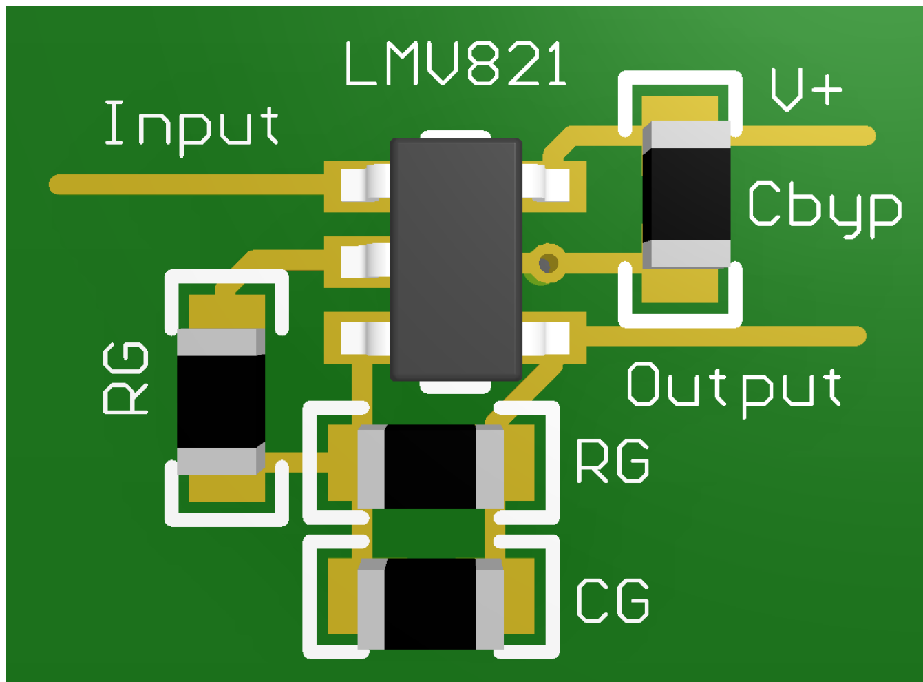
图 48. 3D 布局
