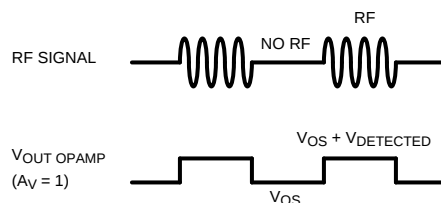
Figure 43. 由于干扰射频信号而导致的偏移电压变化
