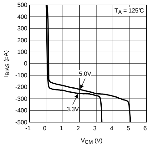
Figure 8. 125^\circ\text{C} 下输入偏置电流与 V_{\text{CM}} 间的关系
