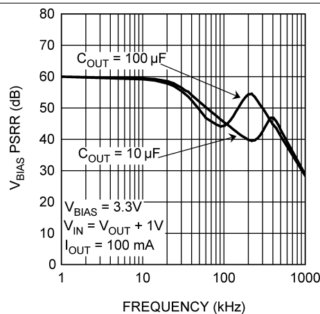
Figure 16. V_{BIAS} PSRR
