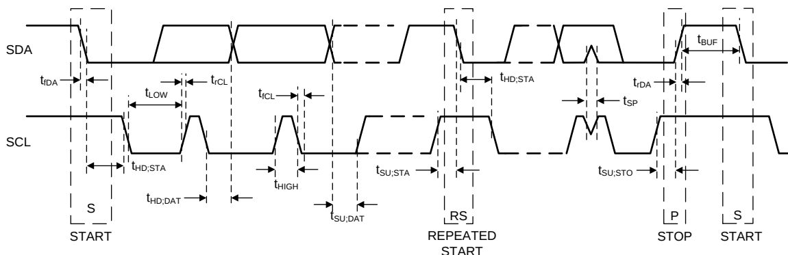
图 18. I²C-Compatible Timing
