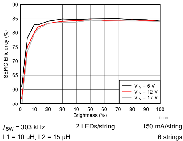
图 6-4. SEPIC Efficiency
