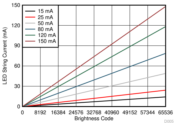
图 6-6. Current Linearity
