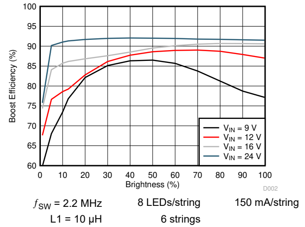
图 6-3. Boost Efficiency
