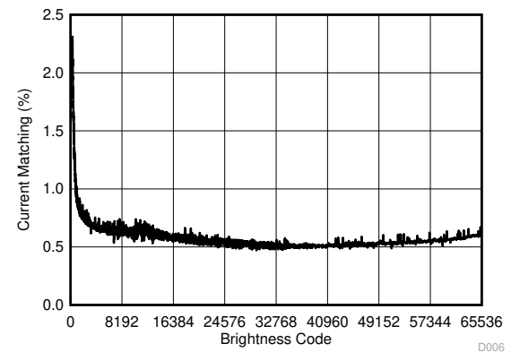
图 6-7. Current Matching
