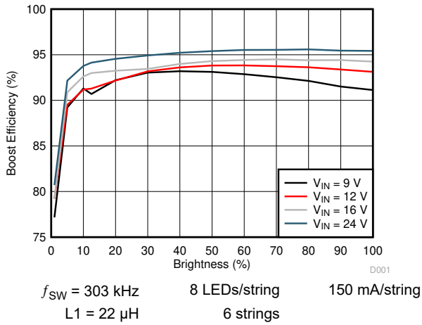
图 6-2. Boost Efficiency
