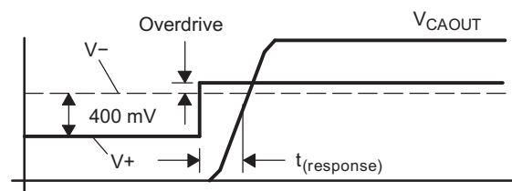
图 33. 过驱的定义
