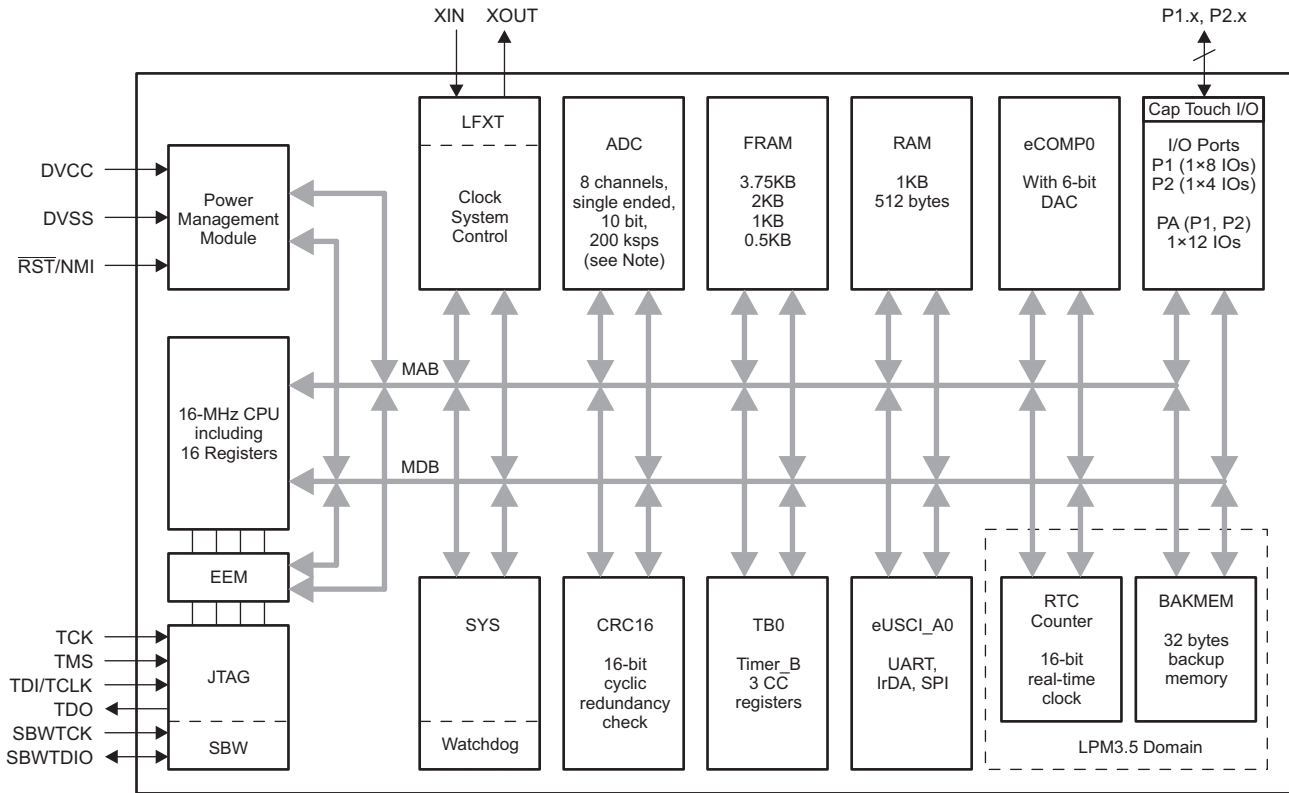
图 1-1. 功能框图
