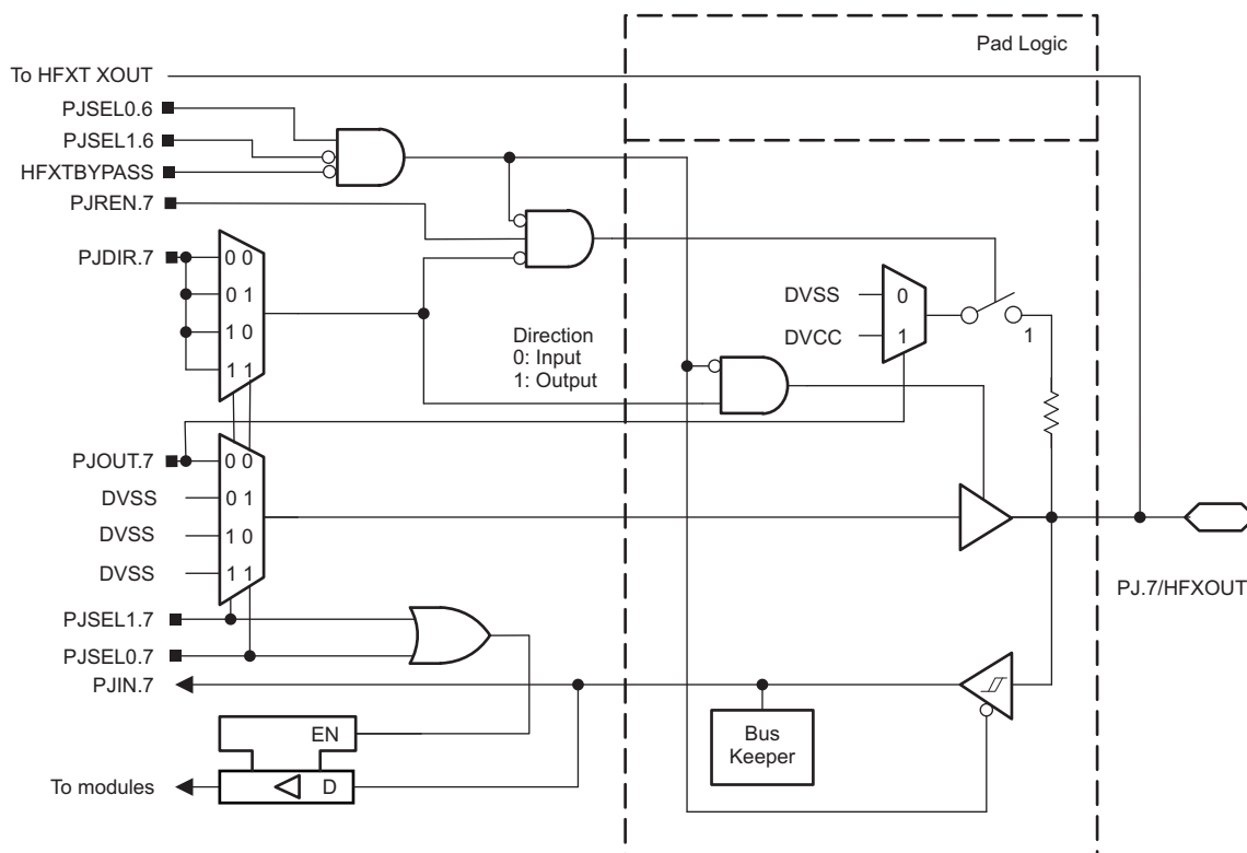
图 6-13. Port PJ (PJ.7) Diagram
