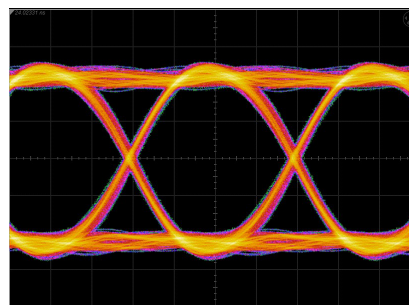
眼图
