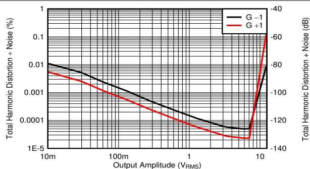
图 6-7. THD+N vs Output Amplitude
