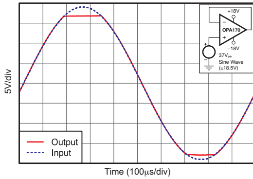
图 25. 无相位反转
