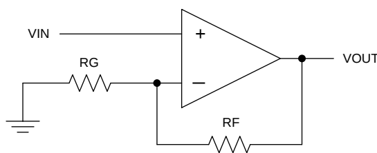
图 44. 原理图表示
