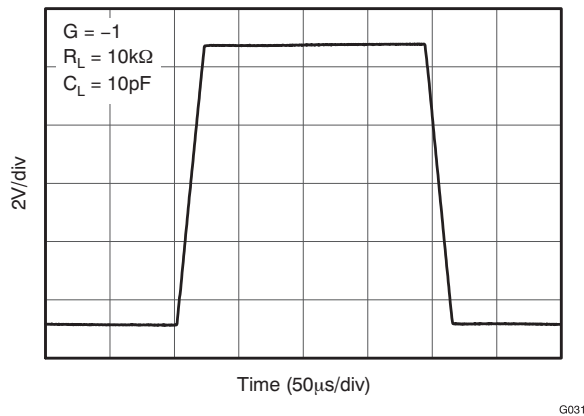
图 31. 大信号阶跃响应
