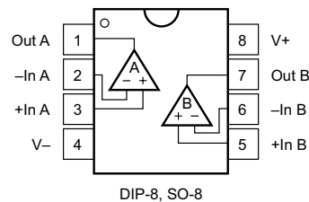
OPA2227、OPA2228: P 或 D 封装 8 引脚 PDIP 或 8 引脚 SOIC 俯视图
