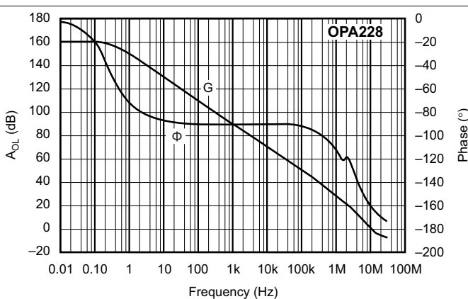
图 2. 开环增益和相位与频率间的关系
