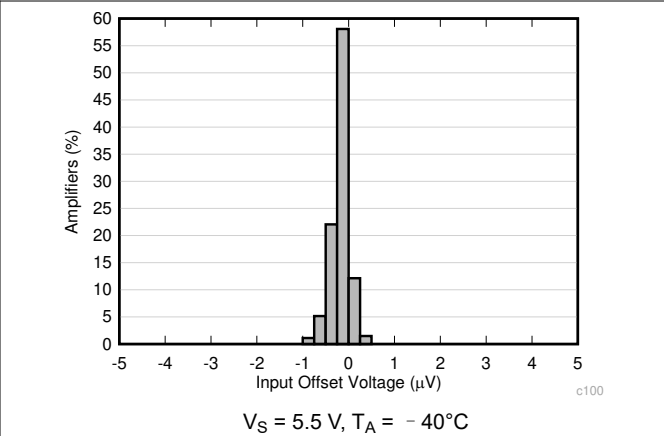
图 6-2. Offset Voltage Distribution
