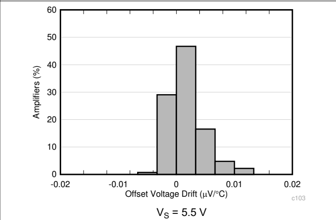
图 6-4. Offset Voltage Drift Distribution
