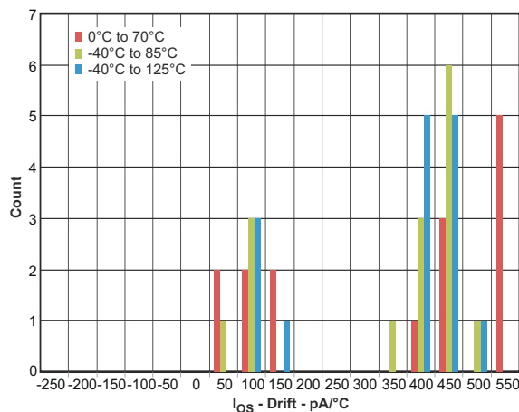
图 7-26. Input Offset Current Drift
