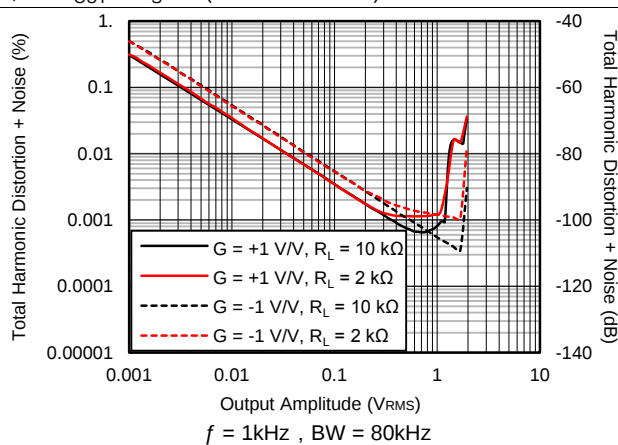
Figure 20. THD + N 与幅度间的关系
