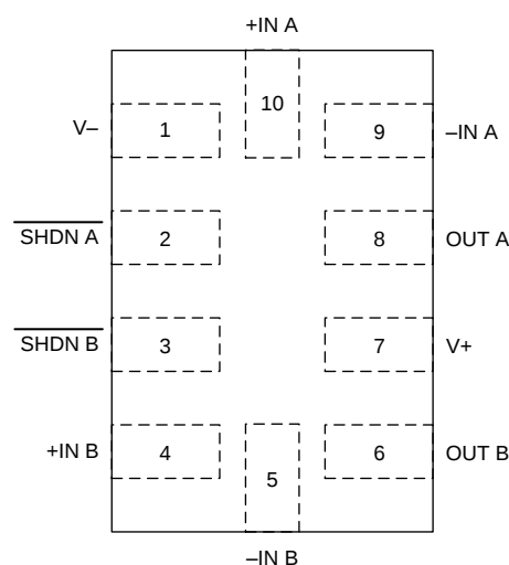
RUG 封装 10 引脚 QFN 俯视图
