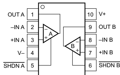
DGS 封装 10 引脚 MSOP 俯视图
