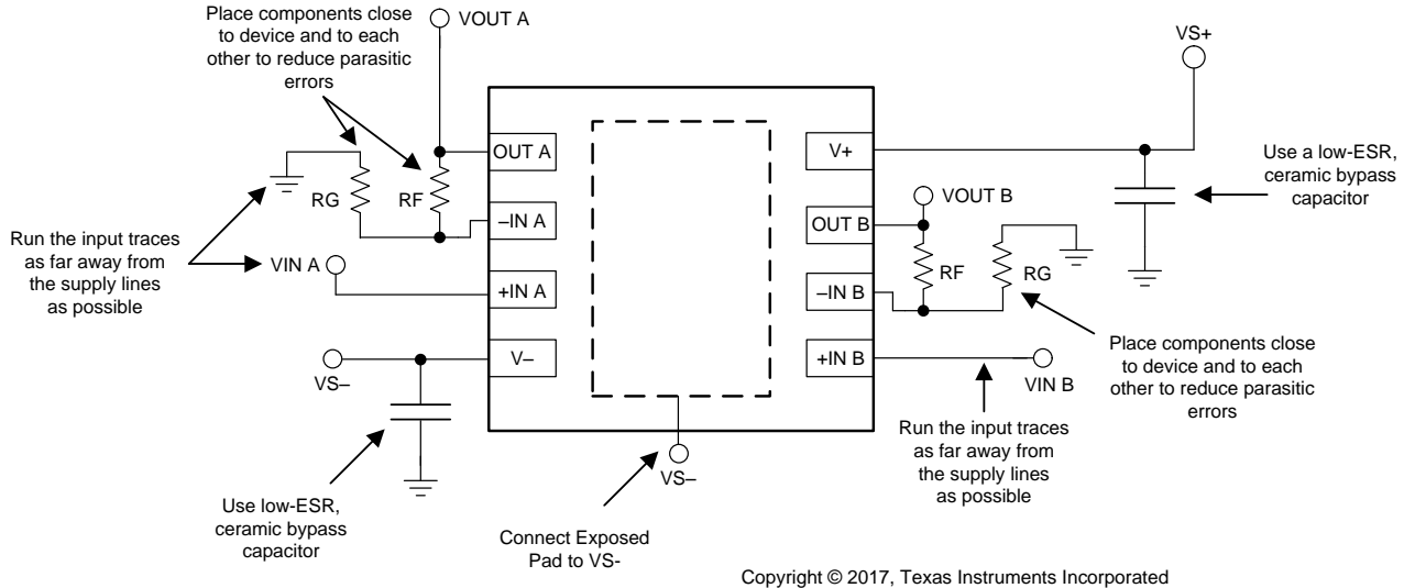
图 29. Layout Example
