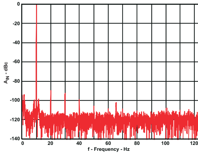
图 9-10. ADS8326 and OPA835 10-kHz FFT
