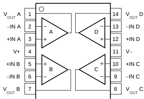
OPA4364 : D 和 PW 封装 14 引脚 SOIC 和 TSSOP 俯视图
