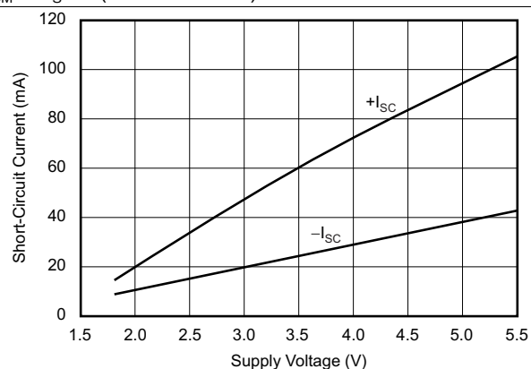
Figure 8. 短路电流与电源电压间的关系
