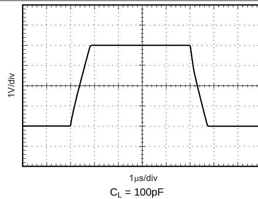
Figure 20. 大信号阶跃响应
