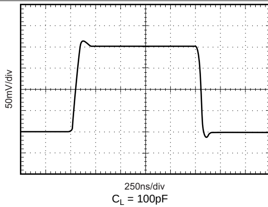
Figure 19. 小信号阶跃响应
