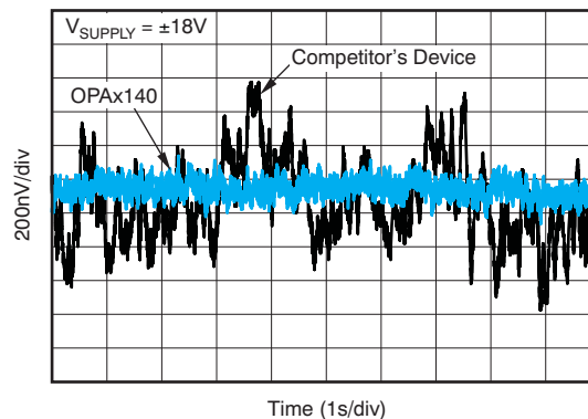
0.1Hz 至 10Hz 噪声
