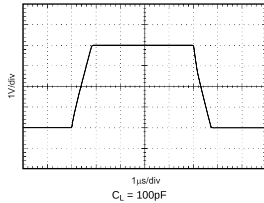
Figure 20. 大信号阶跃响应
