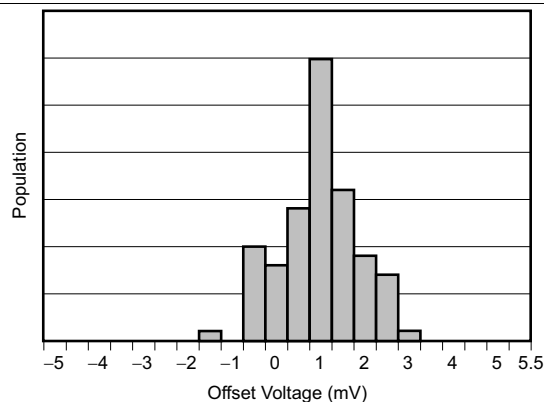
图 14. 失调电压产生分布
