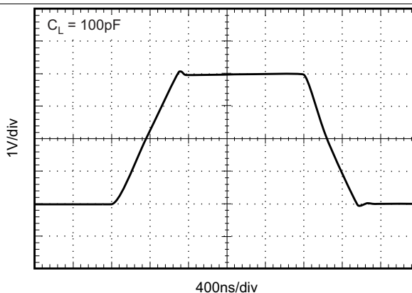
图 18. 大信号阶跃响应
