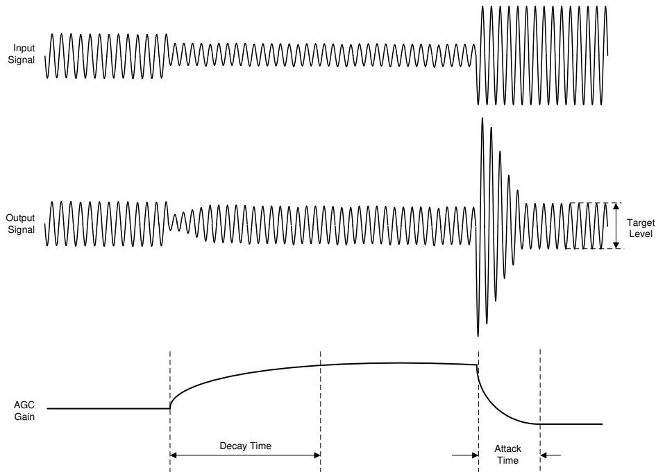
图 8-63. AGC Characteristics
