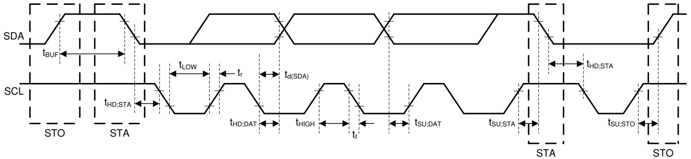
图 7-1. I 2 C Interface Timing Diagram
