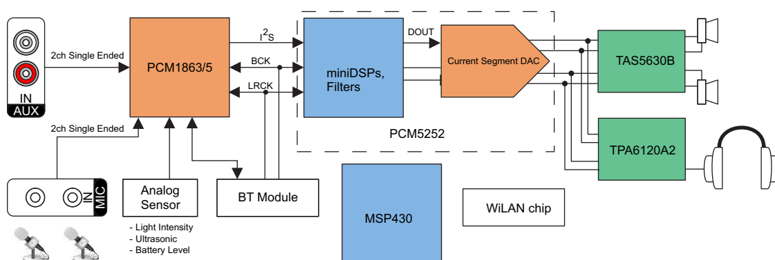
简化系统图
