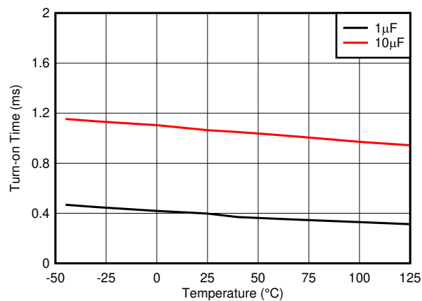
图 10-4. REF70 Turn-on Time
