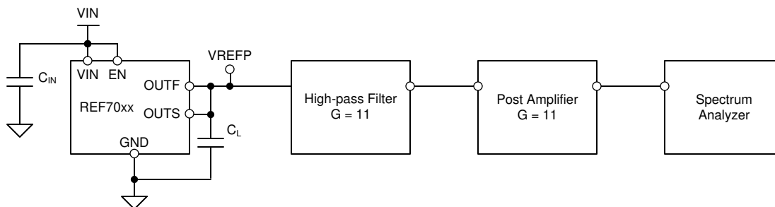
图 8-9. Broadband Noise Test Setup
