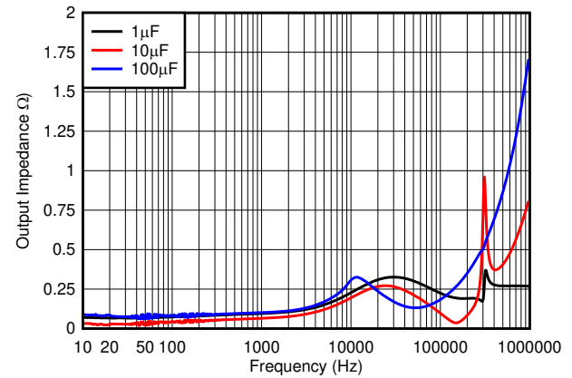
图 7-10. Output Impedance
