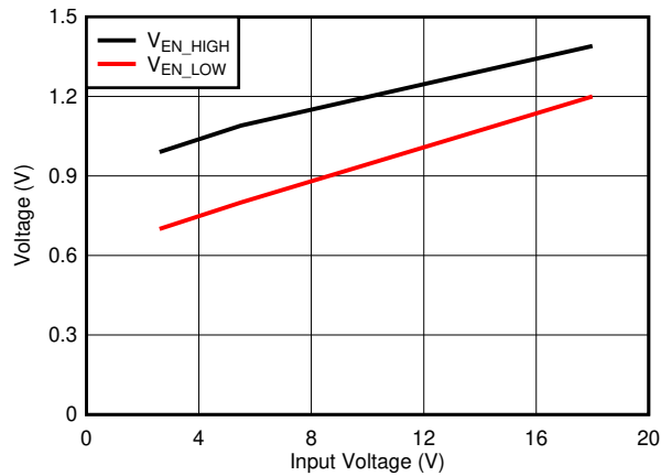
图 7-13. Enable Threshold vs V_{IN}
