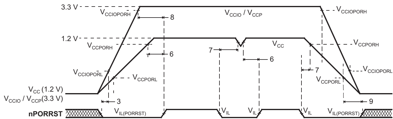
图 5-1. nPORRST 时序图
