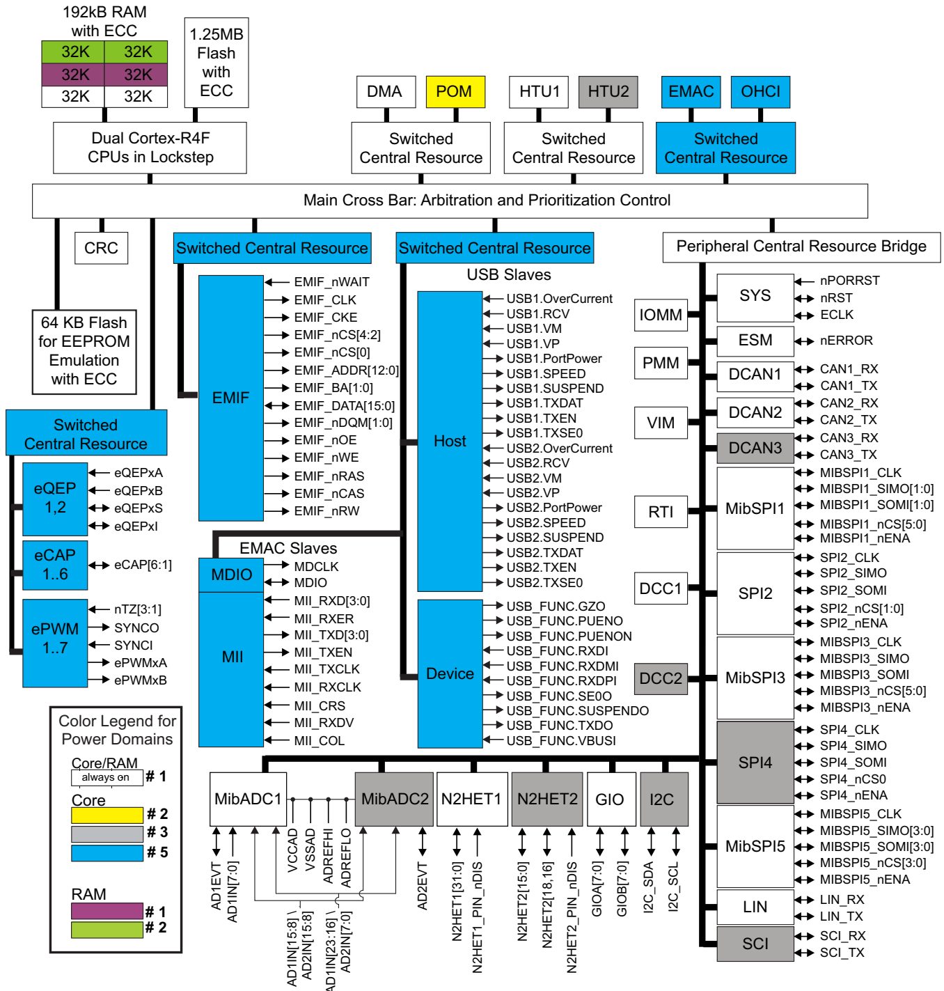
图 1-1. 功能方框图
