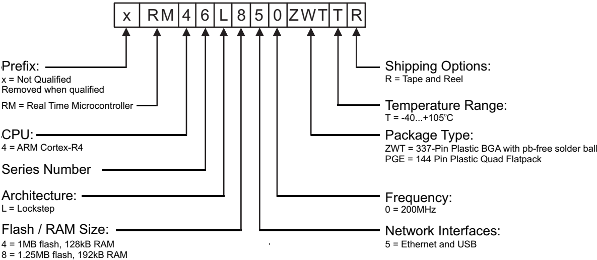
图 7-1. RM46Lx50 器件编号惯例
