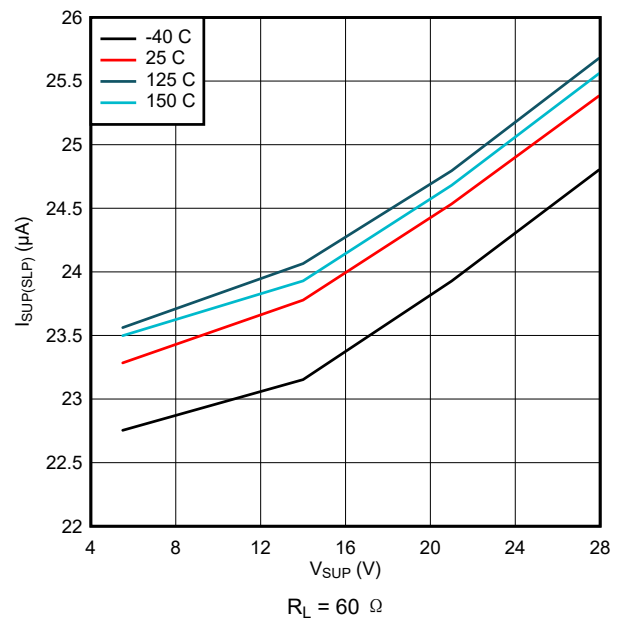
图 7-2. I_{\text{SUP}} over V_{\text{SUP}} Sleep Mode
