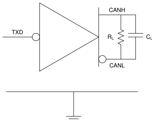
图 8-1. I_{SUP} Test Circuit
