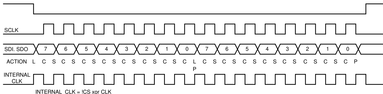
图 9-21. SPI Clocking
