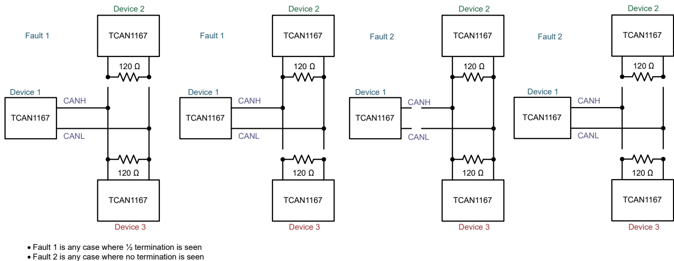
图 9-9. Fault 1 and 2 Examples
