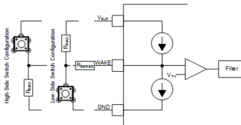
图 9-16. WAKE Circuit Example
