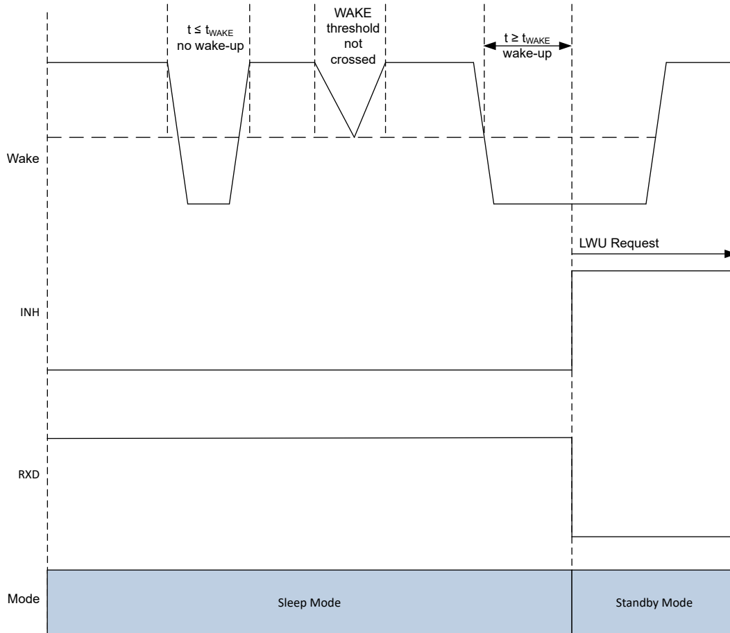
图 9-18. LWU Request Falling Edge
