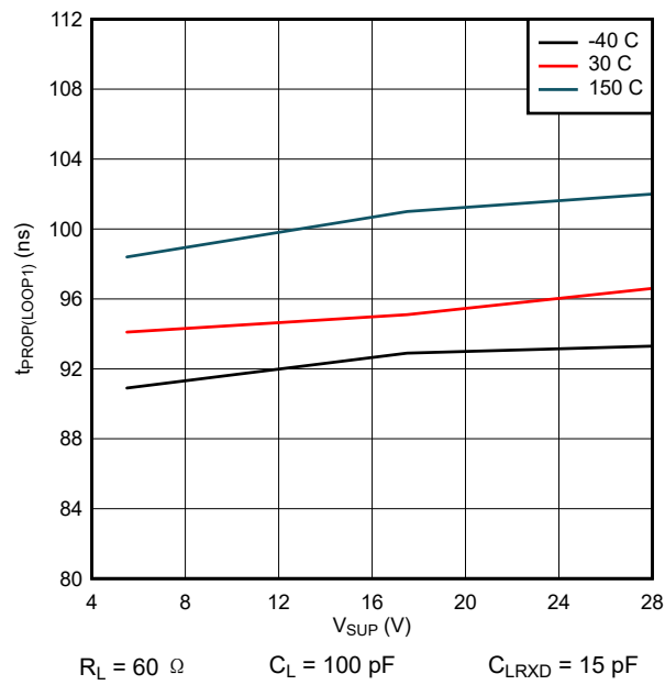
图 7-1. t_{\text{PROP(LOOP1)}} over V_{\text{SUP}}
