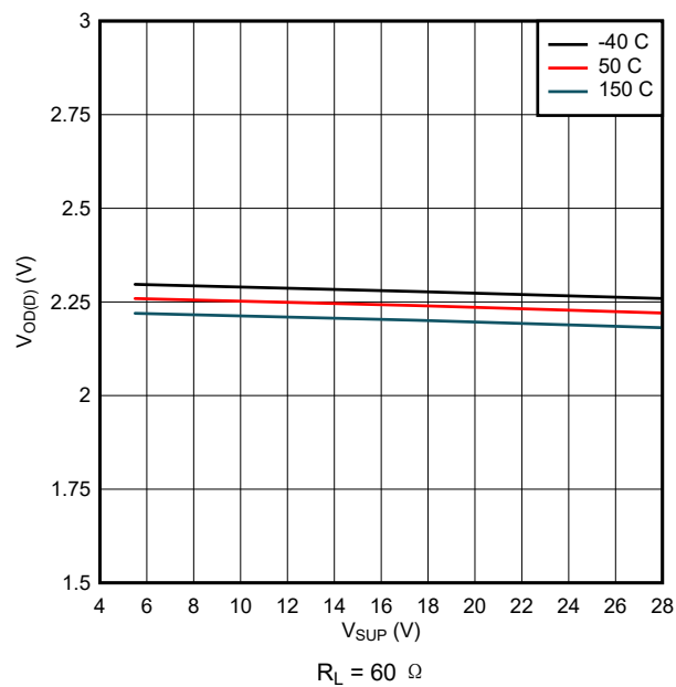
图 7-3. V_{\text{OD(DOM)}} over V_{\text{SUP}}
