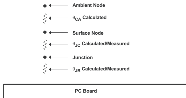
图 11-2. Thermal Resistance
