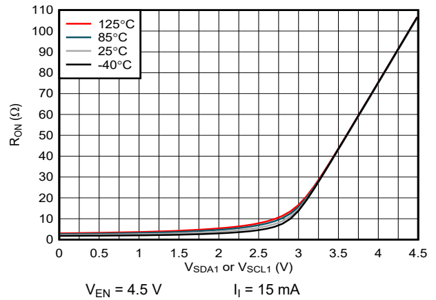
图 6-2. On-Resistance ( R_{ON} ) vs Input Voltage ( V_{SDA1} or V_{SCL1} )
