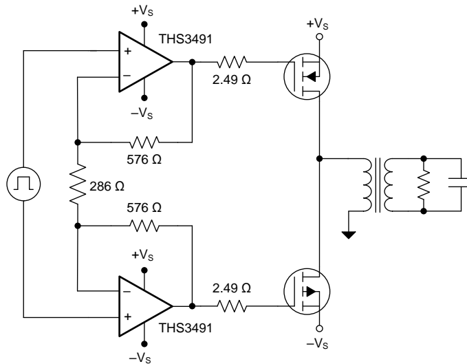
图 67. Power FET Drive Circuit
