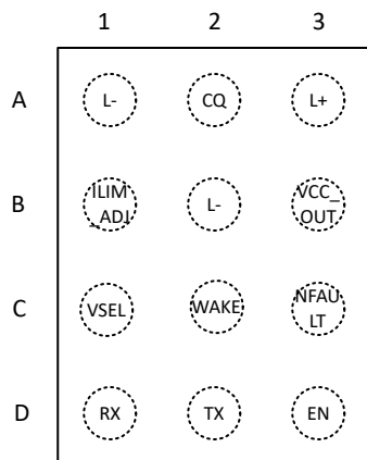
图 5-3. TIOL1123 YAH (DSBGA), 12-Pin (Top View)
