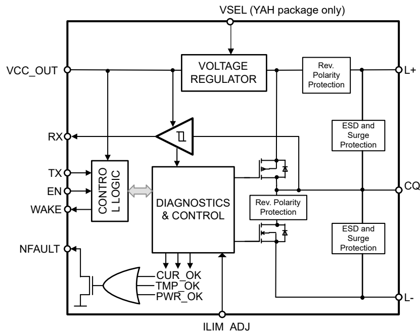
图 8-2. Block Diagram TIOL1123, TIOL1125
