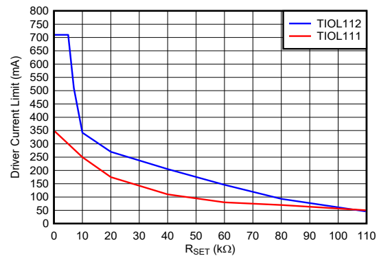
图 6-4. Current Limit vs R_{SET}
