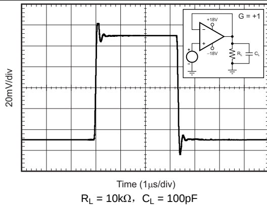
图 17. 小信号阶跃响应 (100mV)
