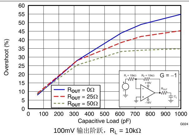
图 15. 小信号过冲与容性负载间的关系
