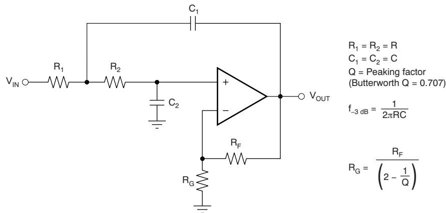
图 30. 两极低通 Sallen-Key 滤波器
