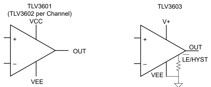
功能方框图
